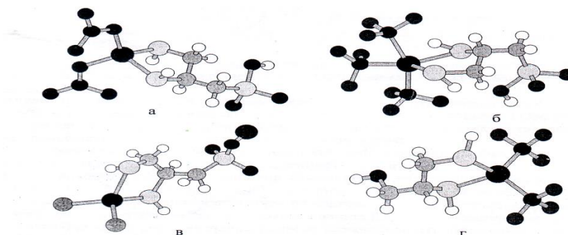
1 сурет – Түрлі лигандалары: а – ДМПСК – М (NO 3 ) 2 ; б – ДМПСК – М (NO 3 ) 3 ; в – Un – MCl 2 ; г – БАЛ – М (NO 3 ) 2 бар металл молекулаларының (II) (Sn, Pb, Hg) және (III) (Tl) геометриялық модельдері.
