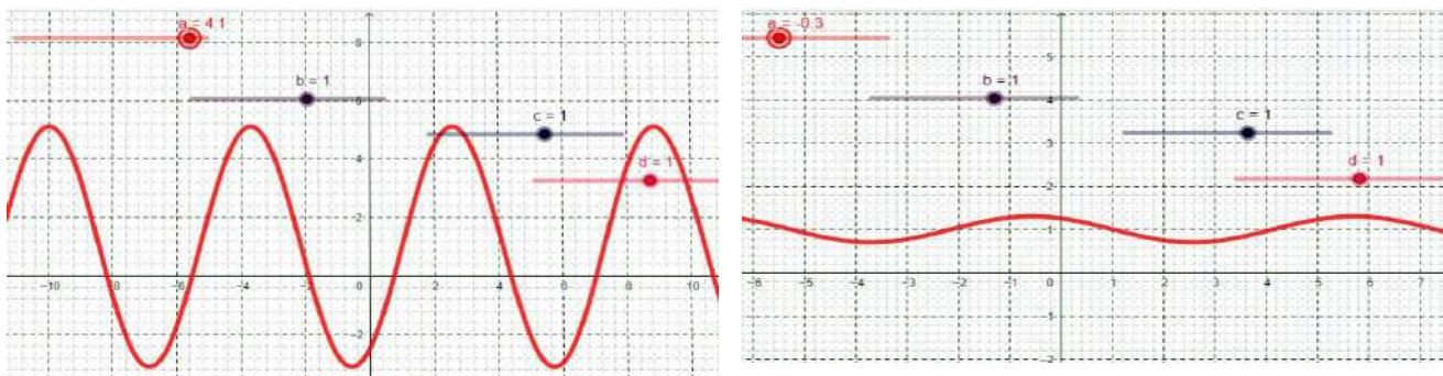
Сурет 6. \sin x функциясы графигінің a мәні бойынша өзгерісі
