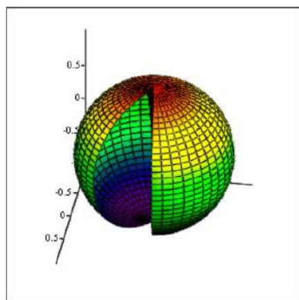
Сурет 5. Координаталарды аналитикалық түрлендіруді пайдалану арқылы алынған ойығы бар шардың графигі
