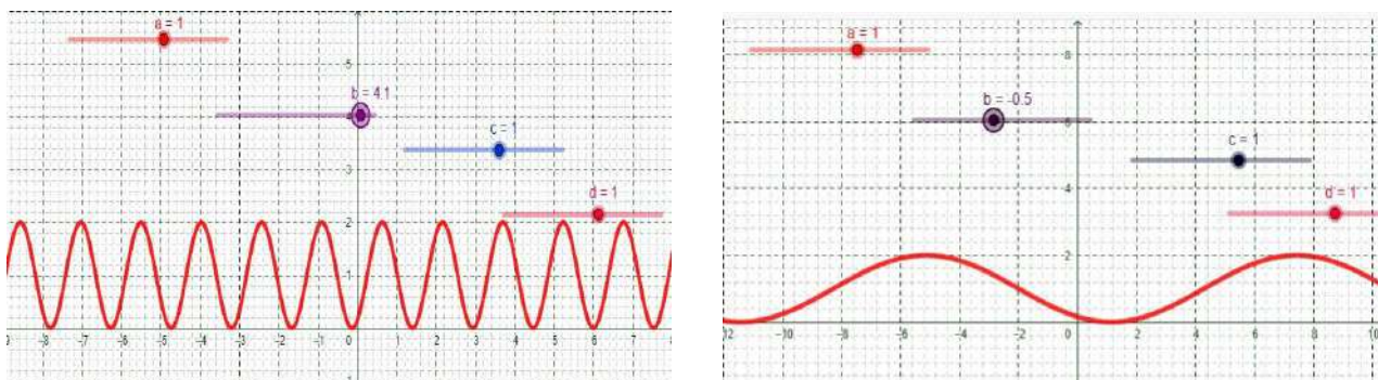
Сурет 7. b мәні өзгерісіне байланысты график кескіні
