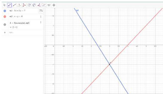
Сурет 2. Функцияның графигі, қиылысу нүктесі мен шешімі
