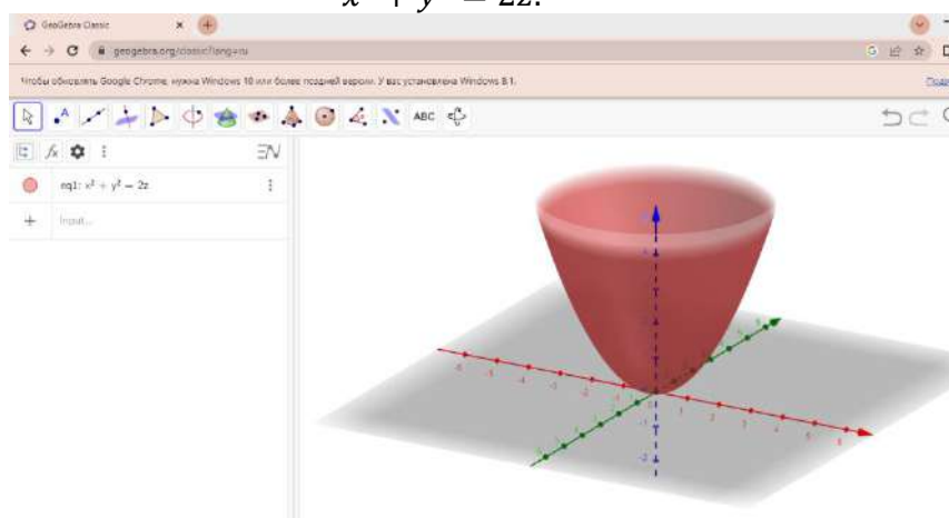
Сурет 8. Эллиптикалық параболоид
