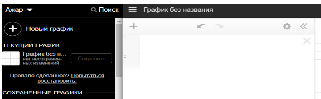
Сурет 6. “Новый график”
