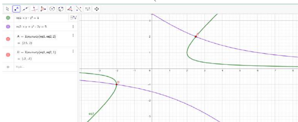
Сурет 3. Тендеулер жүйесінің графигі мен қиылысу нүктелері
