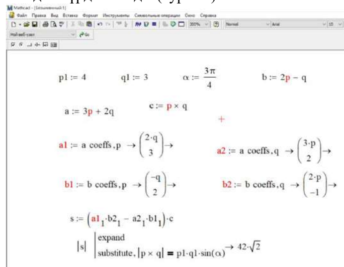
Сурет 2. Векторлардан құралған параллелограмның ауданын есептеу
