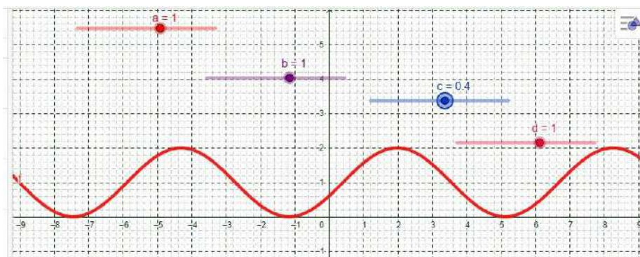
Сурет 8. c мәніне байланысты өзгерісі
