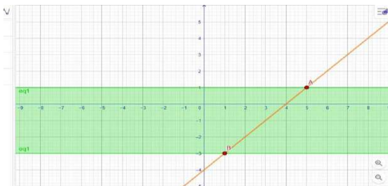
Сурет 4. Графигі мен қиылысу нүктелері
