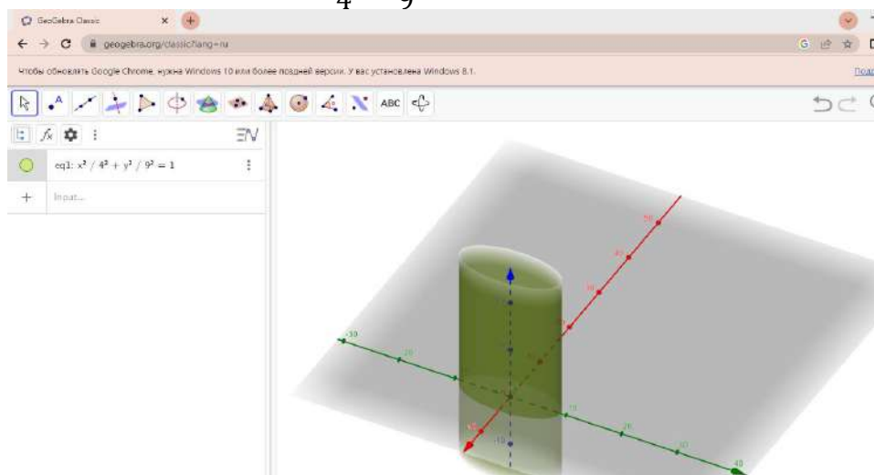
Сурет 4. Эллиптикалық цилиндр
