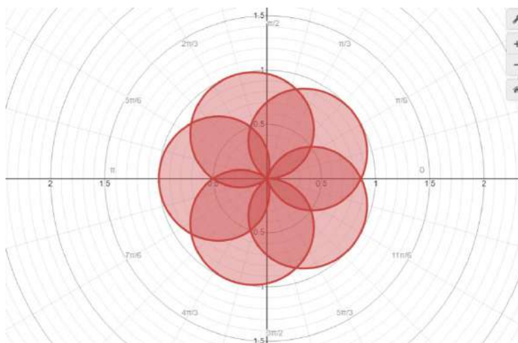
Сурет 10. Полярлық координата: полярлық роза.
