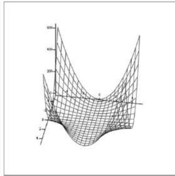
Сурет 3. f(x, y) = x^2 \cdot y^2 функциясының графигі
