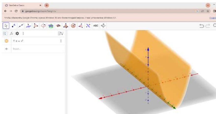
Сурет 5. Параболалық цилиндр
