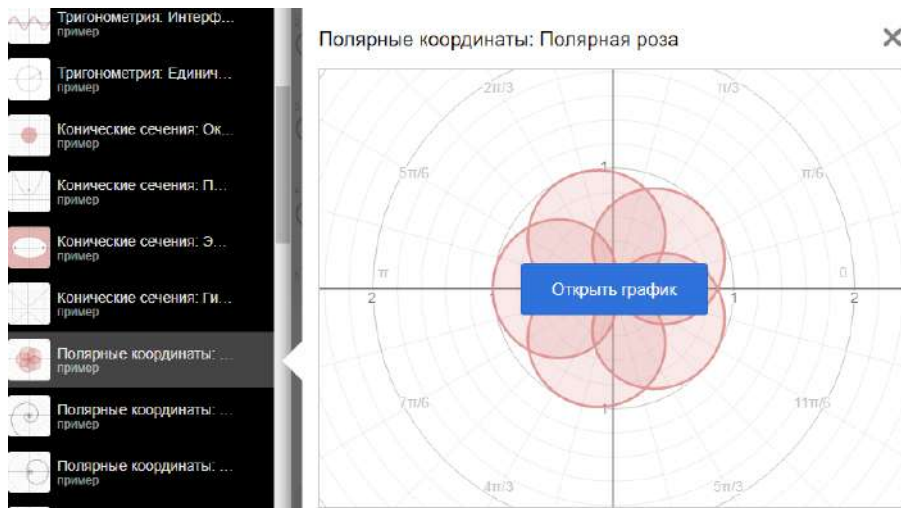
Сурет 8. “Полярная роза” атты мысал
