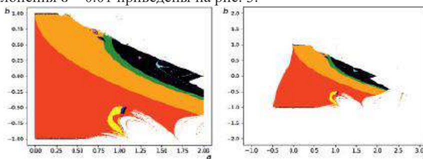
Рис. 3. Карты динамических режимов отображения Эно
