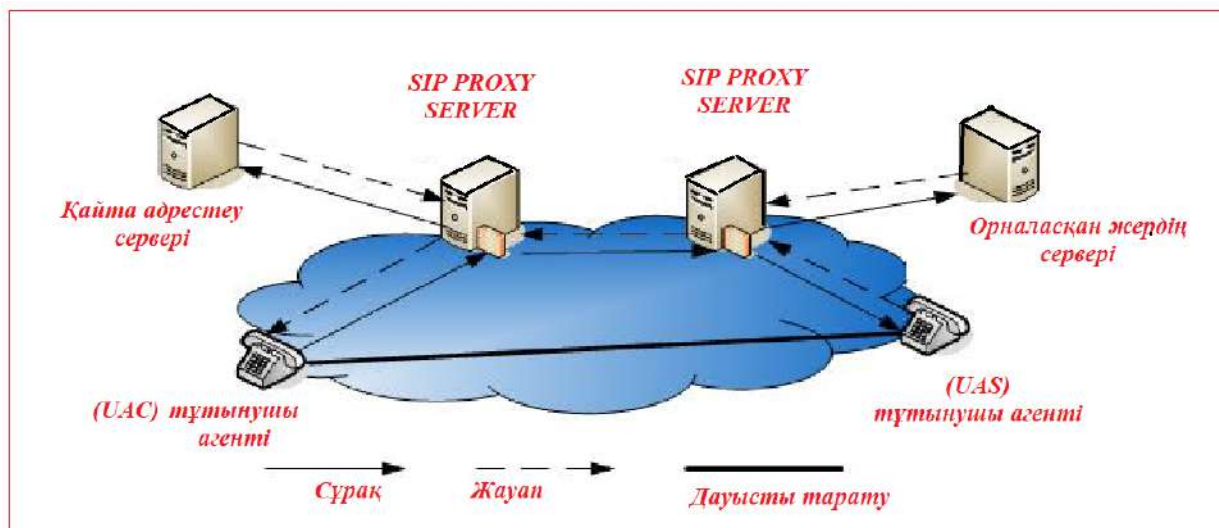
Сурет 2. SIP протоколына негізделген желі мысалы
