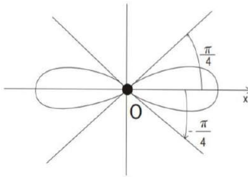
«5-сурет – Бернулли лимнискатасы»
