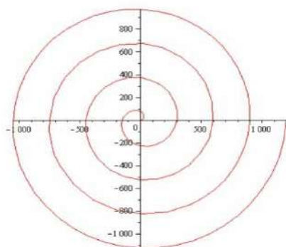
« 3- сурет- plot3d командасы арқылы салынған сызба»
