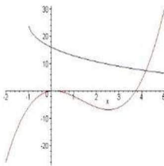
«1 – сурет - plot командасы арқылы алынған сызба»
