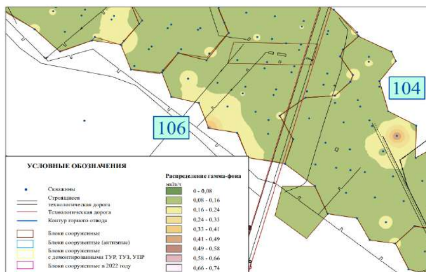
Рисунок 4. Результаты гамма-съемки.
