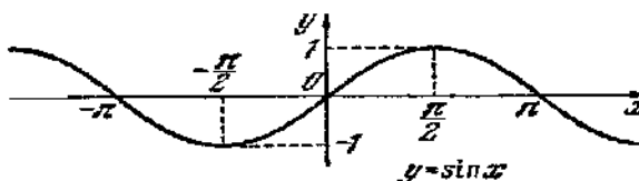
Сурет 1.2 y = \sin x функциясының графигі.
